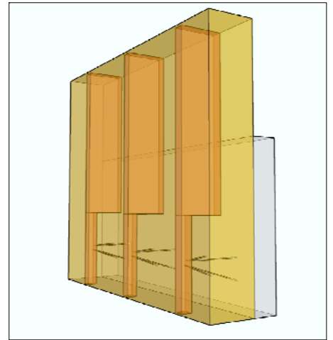
Perspective acrotère M:1/10
