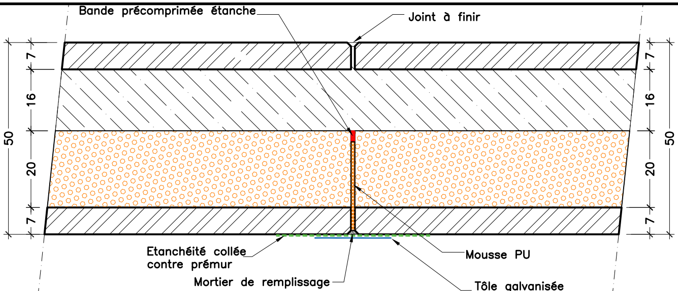
Coupe horizontale
