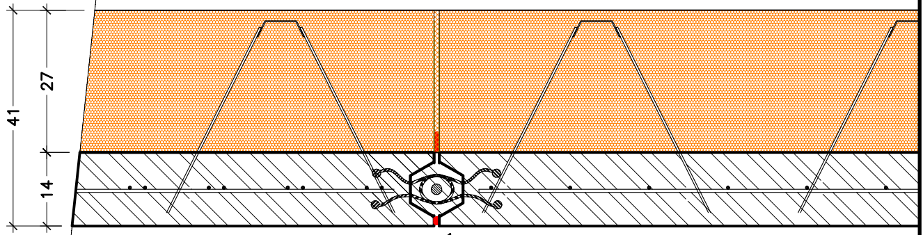
Coupe horizontale
